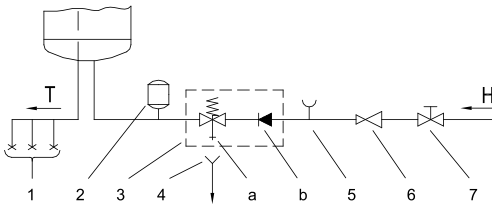
Sl. 3: Zatvoreni (tlačni) sustav
