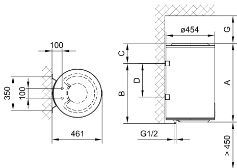
Sl. 1: Vertikalno montiranje na zid
