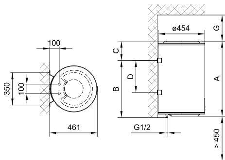
Sl. 1: Uspravno postavljanje na zid
