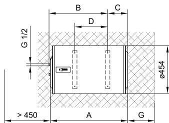
Abb. 2: Waagerechte Montage an die Wand
