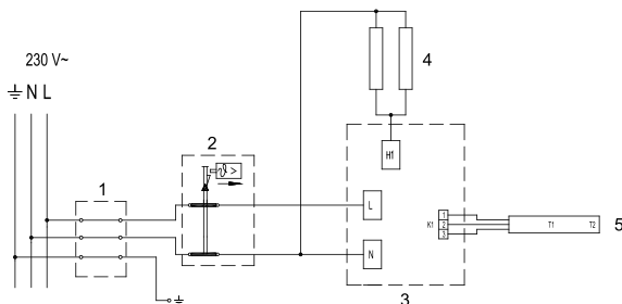
Abb. 6: Elektroschaltbild
