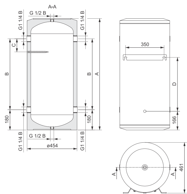
Priključne in montažne mere stenske izvedbe zalogovnika (mm)
