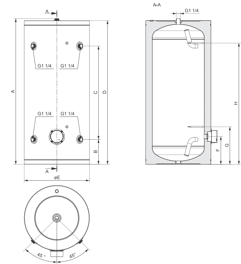
Priključne in montažne mere talne izvedbe zalogovnika (mm)
